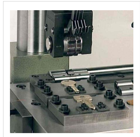
Werkstückspezifische Vorrichtungen
